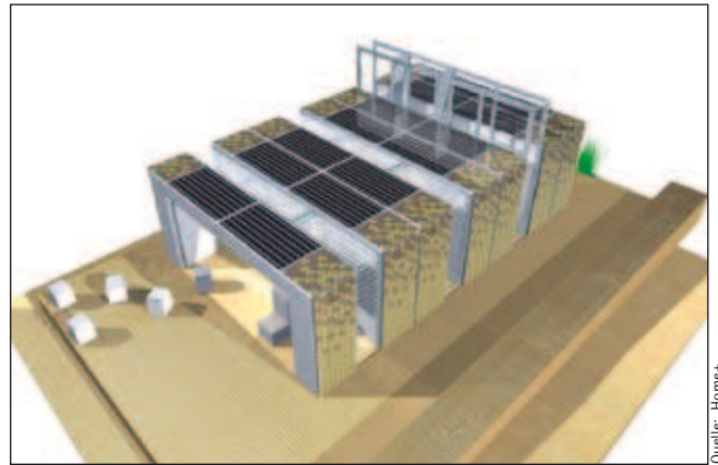
Bild 6: Dauchaufsicht des Home+ der HFT Stuttgart
