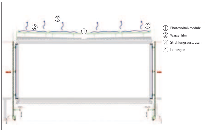
Bild 3: Schnitt durch das Rosenheimer Solarhaus
