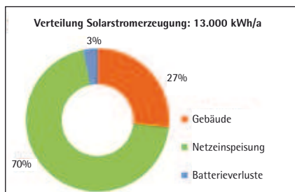
Bild 8: Verteilung des am Gebäude erzeugten Solarstroms für den Standort Madrid
